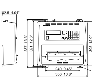
FAX-408 Empfangseinheit 5.6 kg 12.3 lb
