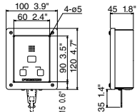
FELCOM250/500 Rufeingangsanzeige FB-3000
