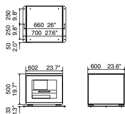
19 inch Rack Gewicht: TBD
