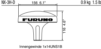
Antenne NX-3H-D 0.9 kg 1.5 lb
