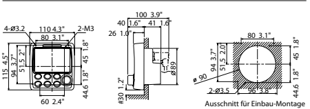
NAVpilot-711 Steuereinheit (Einbau-Montage) 0.35 kg 0.77 lb
