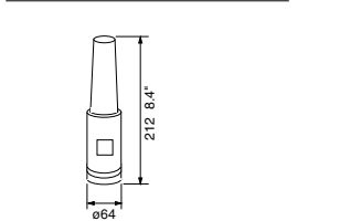
Vorverstärker FAX-5 1.3 kg 2.9 lb
