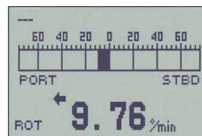
Drehrate (ROT)
