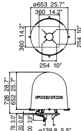
FELCOM500 Antenne FB-1500 21 kg 46.3 lb
