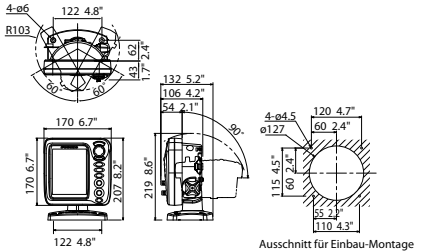
FCV-585 Display Bügelmontage 2.2 kg 4.9 lb Einbau-Montage 1.5 kg 3.3 lb
