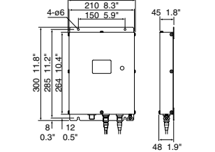
Vorverstärker FAX-5 1.3 kg 2.9 lb
