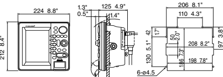
7" LCD (Einbau-Montage)
