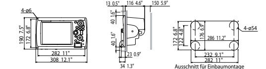
Multifunktions-Display (Einbau-Montage) MFD12 5.4 kg 11.9 lb
