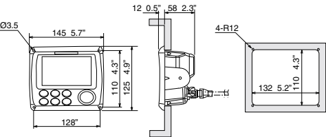
RD-33 Display (Einbau-Montage) 0.6 kg 1.3lb
