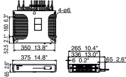
FELCOM250/500 Zentraleinheit FB-2000 4.1 kg 9 lb
