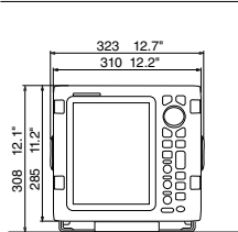
MODELL 1835/1935/1945/1937 Display
