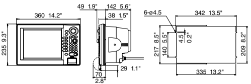
10.4" LCD (Einbau-Montage)
