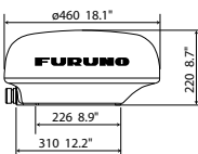
MODELL 1715 Antenne
