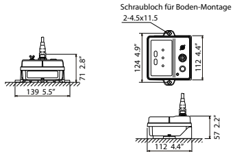
PG-700 (Boden-Montage) Hauptgerät 0.31 kg 0.7 lb
