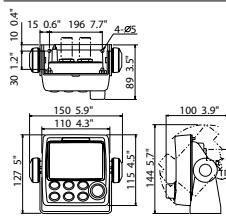
NAVpilot-711 Steuereinheit (Aufbau-Montage) 0.34 kg 0.75 lb
