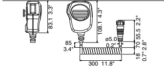
LH-3000 Mikrofon 0.2 kg 0.44 lb
