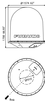
Antenne Gewicht: TBD
