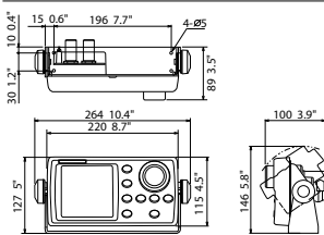
NAVpilot-700 Steuereinheit (Aufbau-Montage) 0.62 kg 1.4 lb
