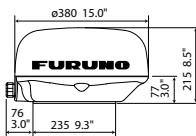
MODELL 1715 Antenne
