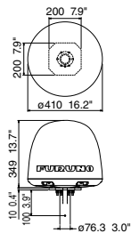
FELCOM250 Antenne FB-1250 6 kg 13.2 lb
