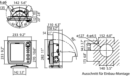
FCV-585 Display Bügelmontage 2.2 kg 4.9 lb Einbau-Montage 1.5 kg 3.3 lb
