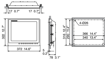
MU-190HD Einbau-Montage 8.0 kg 17.6 lb
