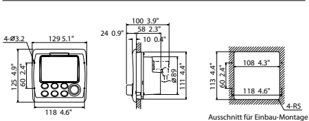
NAVpilot-711 Steuereinheit (Einbau-Montage) 0.35 kg 0.77 lb
