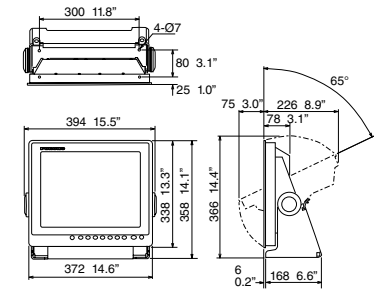
MU-150HD Bügel-Montage 7.0 kg 15.4 lb
