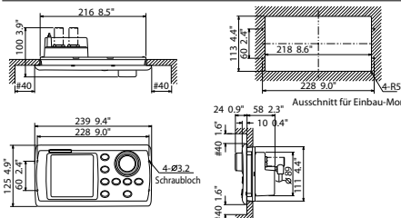
NAVpilot-700 Steuereinheit (Einbau-Montage) 0.64 kg 1.4 lb
