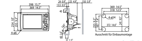
Multifunktions-Display (Einbau-Montage) MFD12 5.4 kg 11.9 lb
