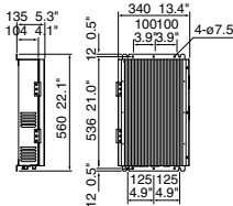
Sende-/Empfangs-Einheit FS-2570T
