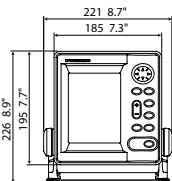
MODELL 1715 Display
