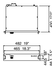
Antenne Steuereinheit Gewicht: TBD
