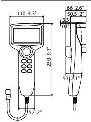
NAVpilot-711 Steuereinheit (Aufbau-Montage) 0.34 kg 0.75 lb
