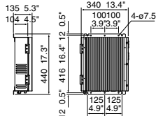
Sende-/Empfangs-Einheit FS-1570T
