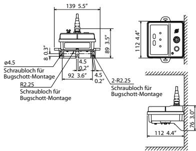
PG-700 (Bugschott-Montage) Hauptgerät 0.35 kg 0.77 lb
