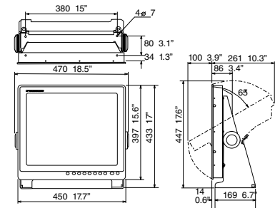
MU-190HD Bügel-Montage 12 kg 26 lb
