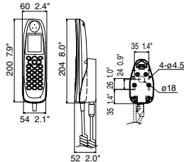
FELCOM250/500 Handset FB-8000 0.38 kg 0.8 lb
