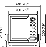
MODELL 1715 Display
